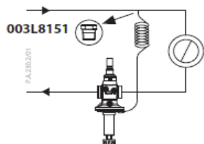
Impulzní trubka připojená na přívodní potrubí
