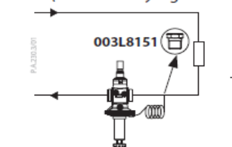
Impulzní trubka připojená na vratné potrubí
