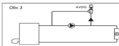
Příklad 2: Regulace přepuštěním přes cirkulační čerpadlo
