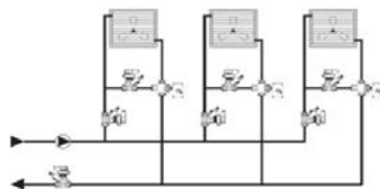
Sekundární okruh pro chlazení nebo vytápění
