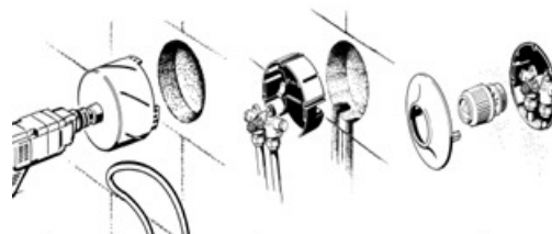
Regulace teploty podlahy u kombinovaného systému topná smyčka s ventilovým tělesem FHV-R ve vratném potrubí.
