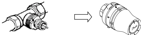
Termostatický ventil RTD-N
