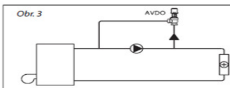
Príklad 2: Regulace prepúštením přes cirkulační čerpadlo
