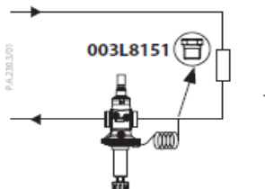
Impulzní trubka připojená na vratné potrubí
