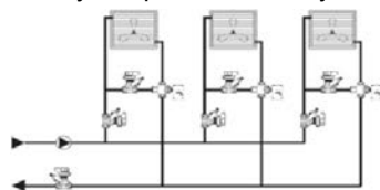
Sekundárny okruh pre chladenie alebo vykurovanie
