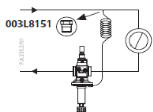
Impulzní trubka připojená na přívodní potrubí
