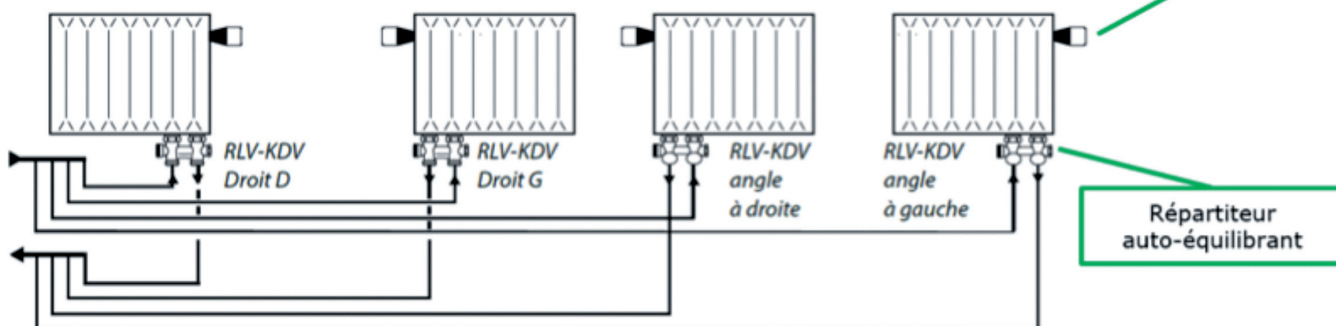
Système bitubes avec radiateurs à robinetterie intégrée, types de raccordement courants.
