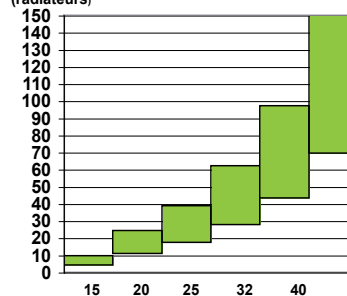
Puissance kW pour DeltaT 15K (radiateurs)
