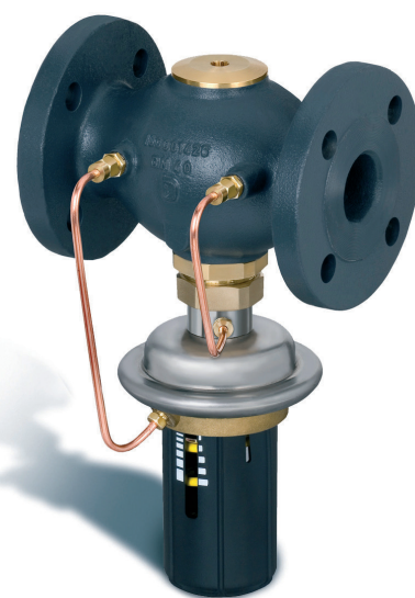
AVPA DN 32 à DN 50 Nous consulter
