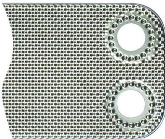
KONŠTRUKCIA NOVÉHO TEPELNÉHO VÝMENNÍKA MICRO PLATE
