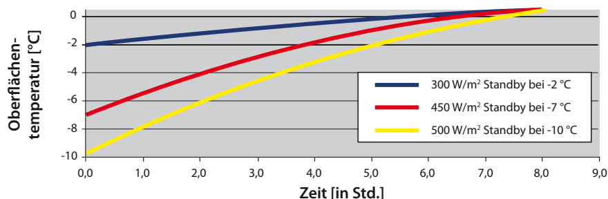
Aufheizzeit für drei Einstellungen der gleichen Auffahrt mit Sandgrund und 80 mm Pflastersteine bei Lufttemperatur von -8°C
