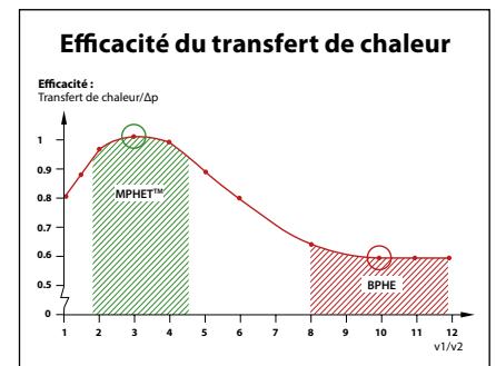
Échangeurs de chaleur MicroPlate™
