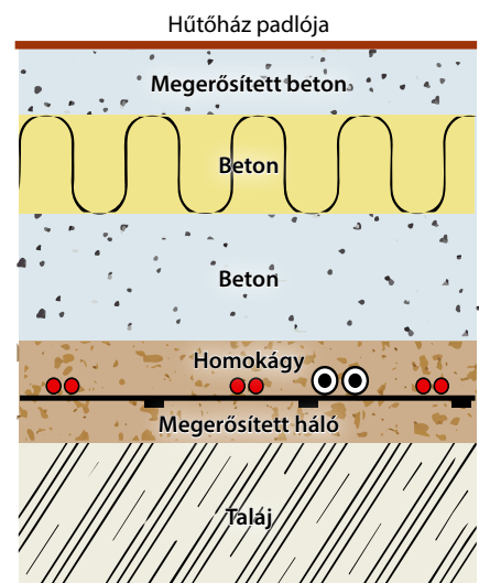
2. ábra – Fűtőkábel a homokágyban
